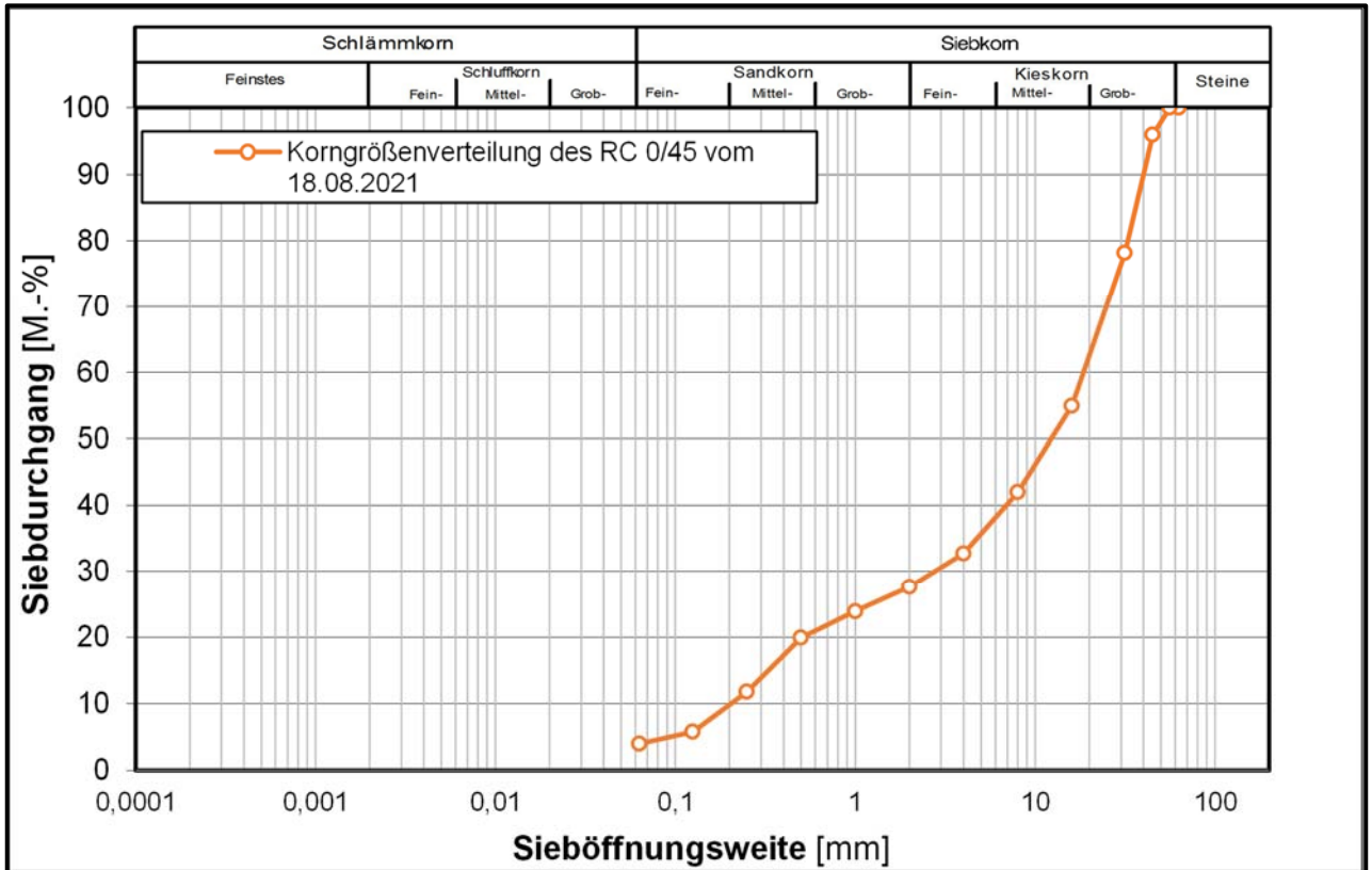
Korngrößenverteilung des untersuchten RC-Materials 0/45
