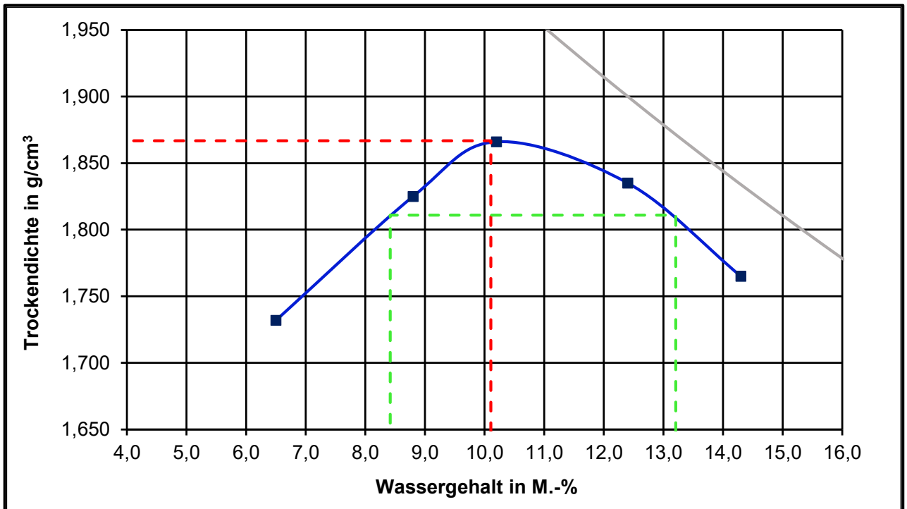
Proctorkurve des untersuchten RC-Materials 0/45 (aus F 21/06/0462)
