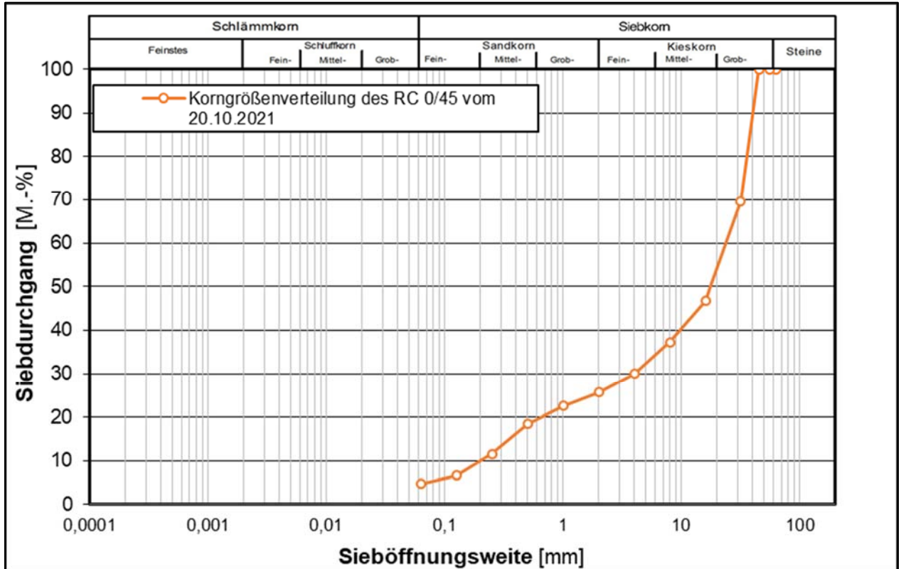
Korngrößenverteilung des untersuchten RC-Materials 0/45
